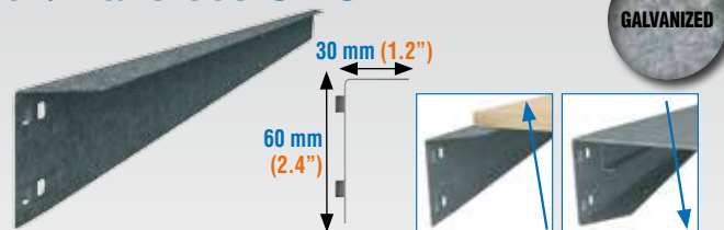
Larguero Serie L95 - Beam L95 Series
