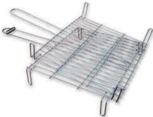
Cod. - 70825 - (25x25 cms.) Cod. - 70830 - (30x30 cms.) Cod. - 70835 - (35x35 cms.) Cod. - 70840 - (40x40 cms.) Cod. - 70845 - (45x45 cms.) Cod. - 70850 - (50x50 cms.) Parrilla Doble Cincada Double Zinc Grill
