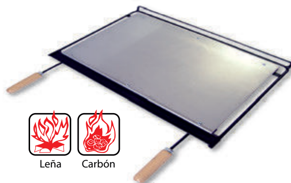
Cod.-71665 - (58x40 cms.) (Para Barbacoas cod.-71406-71407-71550 71552-71554-71556-71558-71561-71563) Cod.-71666 - (68x40 cms.) (Para Barbacoas cod.-71408-71409-71551 71553-71555-71557-71559-71562-71564) Plancha Barbacoa Inox - Steel Barbecue Griddle
