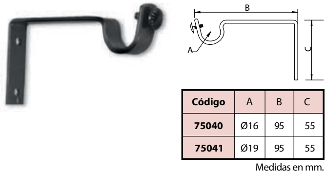
Soporte Doble (para Barra de 16 y 19) - Double Wall Support
