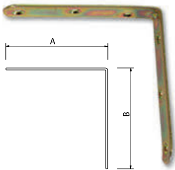
Escuadra Canto Redondo Bicromatada - Flat Corner Iron
