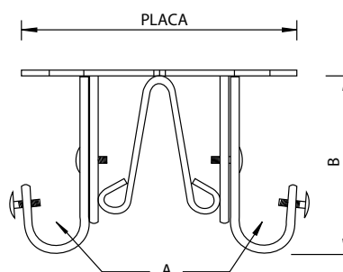
Soporte Techo Doble Extensible (para Barra de 16, 19 y 25) - Double Extending Ceiling Support
