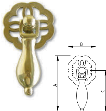
Tirador Péndulo Latón - Brass Handle
