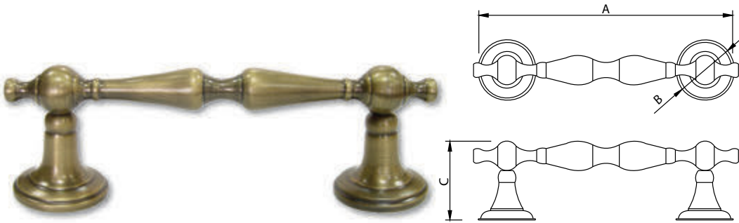
Manillón Latón Patinado - Patinated Brass Handle
