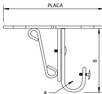
Soporte Techo Doble Extensible (para Barra de 16, 19 y 25) - Double Extending Ceiling Support
