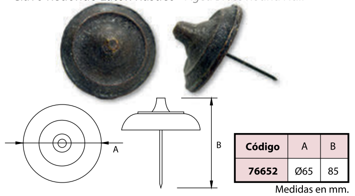
Clavo Latón Rústico - Aged Brass Nail
