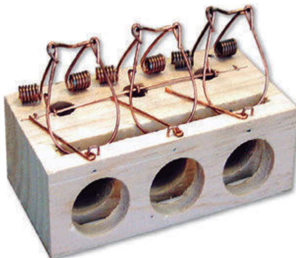
Cod.-40105 - (Ø 28 mm.) Pequeña Cod.-40107 - (Ø 37 mm.) Mediana Cod.-40109 - (Ø 50 mm.) Grande Ratonera 3 - Mouse Trap with 3 Holes
