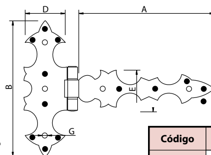
Bisagra Capuchino Estirada - Hinge
