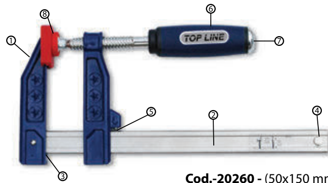
Sargento Reforzado Mango Soft: ① Cuerpo de acero fundido. ② Varilla extra fuerte estriada en ambos lados, forma U. ③ Remache de seguridad en la cabeza. ④ Tope de freno. ⑤ Seguro de fijación antideslizante. ⑥ Mango soft material TPR. ⑦ Remache cromado. ⑧ Protecciones de goma.
