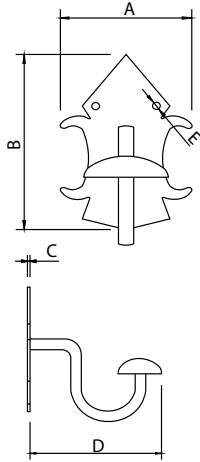
Percha Simple Simple Hook
