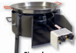
Ejemplo con quemador gas y paellerro
