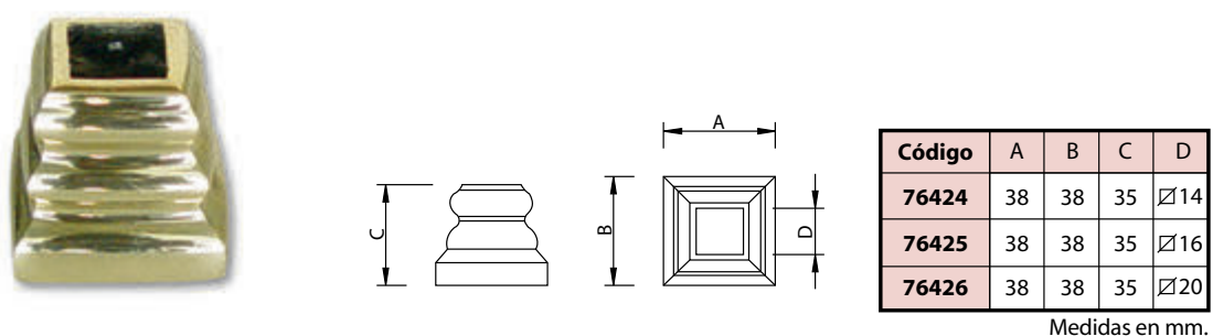
Macolla Base Cuadrado Latón - Brass Decoration for Bars
