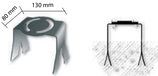
Cod.-11103 - (130x80 mm.) Soporte de Fijación a Hormigón Weather Vane Support
