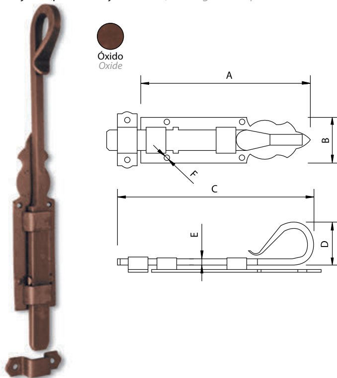
Pasador Forjado (placa 130 y 200 mm.) - Wroght Bolt (plate 130 and 200 mm.)
