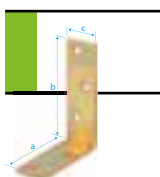
ESCUADRA PARA POSTE DE CARAS DESIGUALES, BICROMATADA JOIST HANGER CONNECTOR, UNEQUAL-SIDED, YELLOW ZINC PLATED ÉQUERRE À POUTRE INÉGALE, BICHROMATÉE
