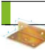
ESCUADRA GRANDE DE CARAS DESIGUALES, BICROMATADA ANGLED BRACKET LARGE, UNEQUAL-SIDED, YELLOW ZINC PLATED ÉQUERRE LARGE, INÉGALE, BICHROMATÉE
