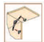
Insertar a presión al compás BCP6 en los enganches de succión rápida, quedando el tornillo de regulación al interior del mueble (nunca al exterior).
