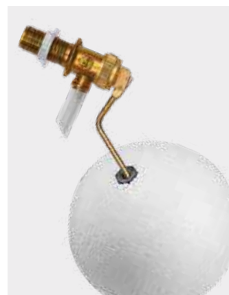
GPB 2 Ref. 0151551530 Packaging Bolsa 25 uds/caja PVP: 8,80 € Grifo lateral (Latón) + Tuerca (Plástico) + Boya Ø 3/8" Latón + Longitud: 32 mm
